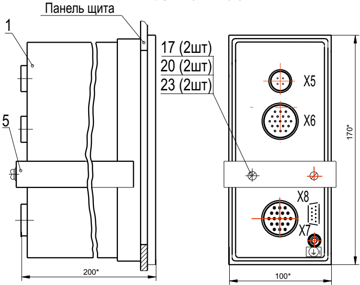
УСТАНОВКА БЛОКА
