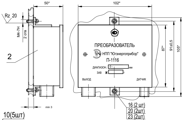
УСТАНОВКА ПРЕОБРАЗОВАТЕЛЯ
